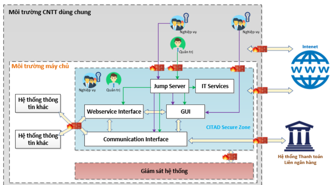
Hình 5: Mô hình tham chiếu an toàn thông tin Hệ thống CITAD
