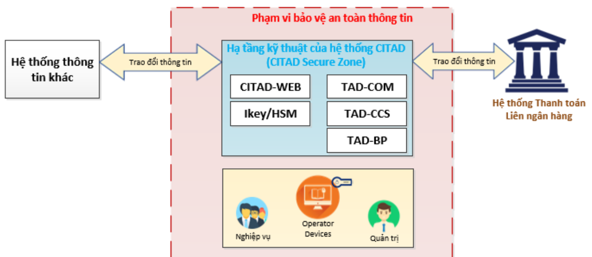
Hình 3: Phạm vi bảo vệ an toàn thông tin Hệ thống CITAD
