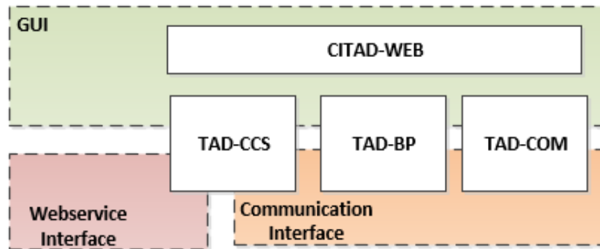
Hình 4: Mô hình tham chiếu giao diện các phần mềm ứng dụng Hệ thống CITAD
